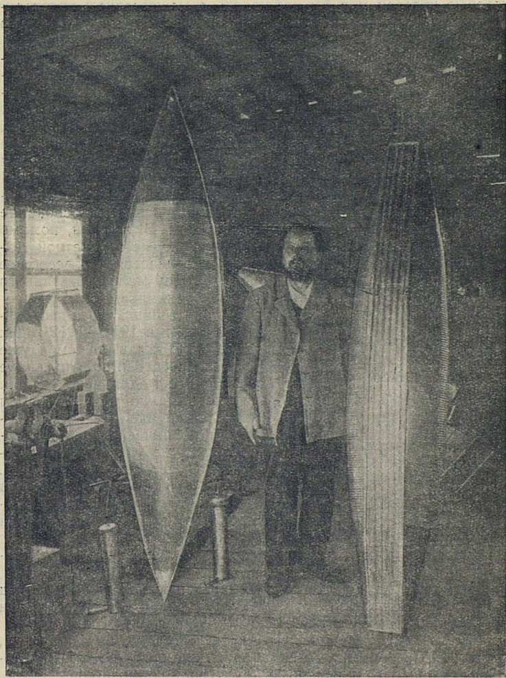
Модели цельнометаллического дирижабля К. Э. Циолковского, изготовленные им собственноручно из жести, которые он показывал на Всероссийском воздухоплавательном съезде в Петербурге в 1914 году.
