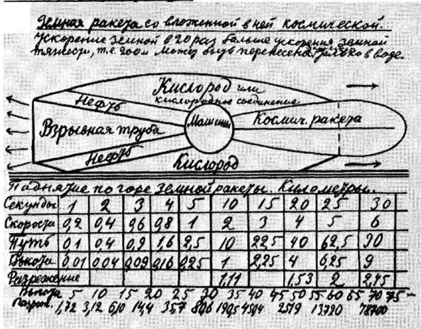
Схема ракеты со вложенной в нее космической ступенью («Альбом космических путешествий»)
